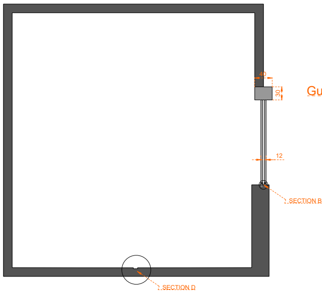
A-A DETAIL
